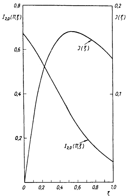
Рис. 1. Зависимость классических орбитальных интегралов I_{2,0}(\pi, \xi) и J(\xi) от параметра адиабатичности \xi
