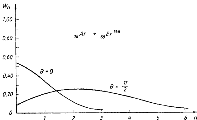
Рис. 3. Вероятность возбуждения n^{20} \beta -вибрационного уровня ядра \text{Er}^{166} при столкновении \text{Ar}^{40} + \text{Er}^{166} ( E \approx V_B ) при C = 60 МэВ. \theta = 0 — вариант А; \theta = \pi/2 — вариант В
