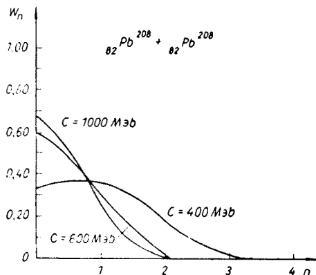
Рис. 2. Вероятность возбуждения n^{20} \beta -вибрационного уровня ядра \text{Pb}^{208} при столкновении \text{Pb}^{208} + \text{Pb}^{208} ( E \approx V_B ) в зависимости от значения параметра жесткости C
