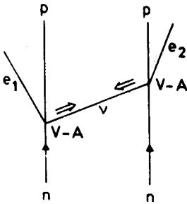
a) m_\nu \neq 0
